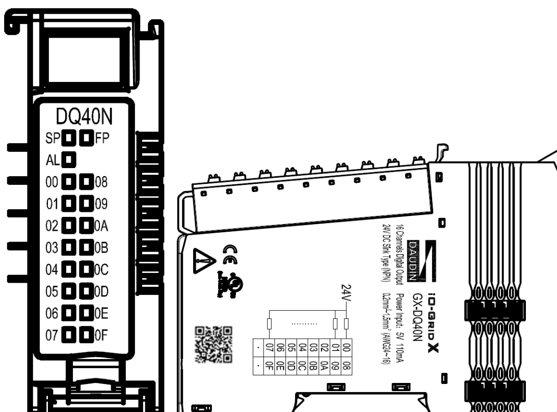
圖 4. 11 GX-DQ40N 圖面
