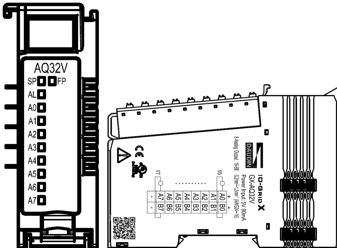
圖 4.31 GX-AQ32V 圖面
