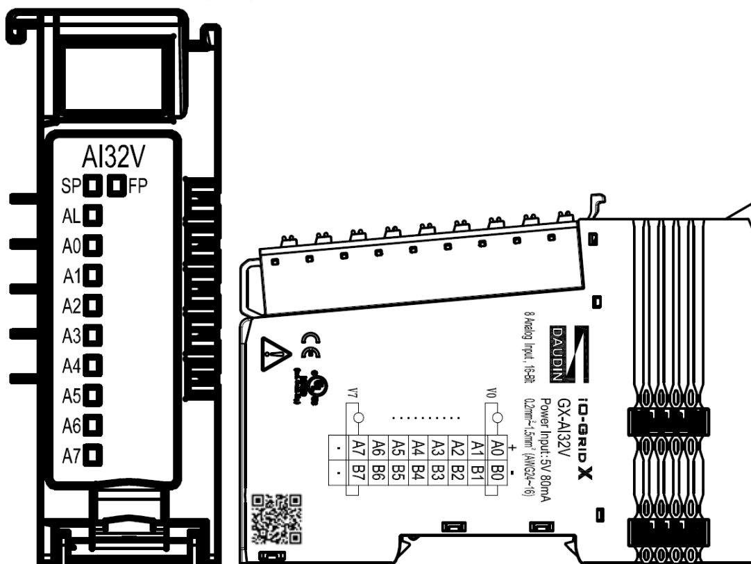
圖 4.23 GX-AI32V 圖面
