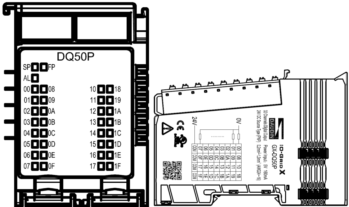
圖 4.14 GX-DQ50P 圖面
