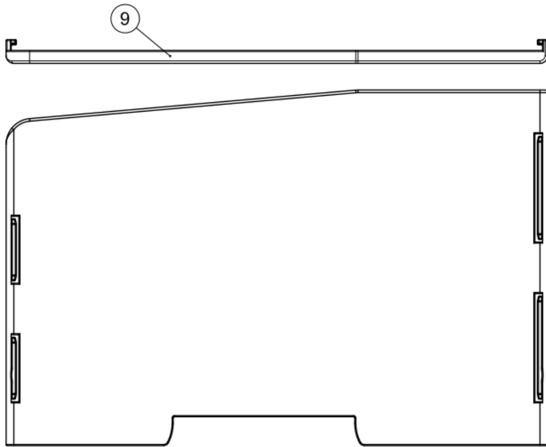
圖 4.1 側面蓋板圖
