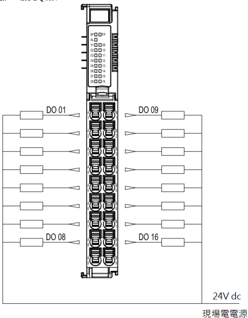
圖 8. 8 GX-DQ40N 接線圖
