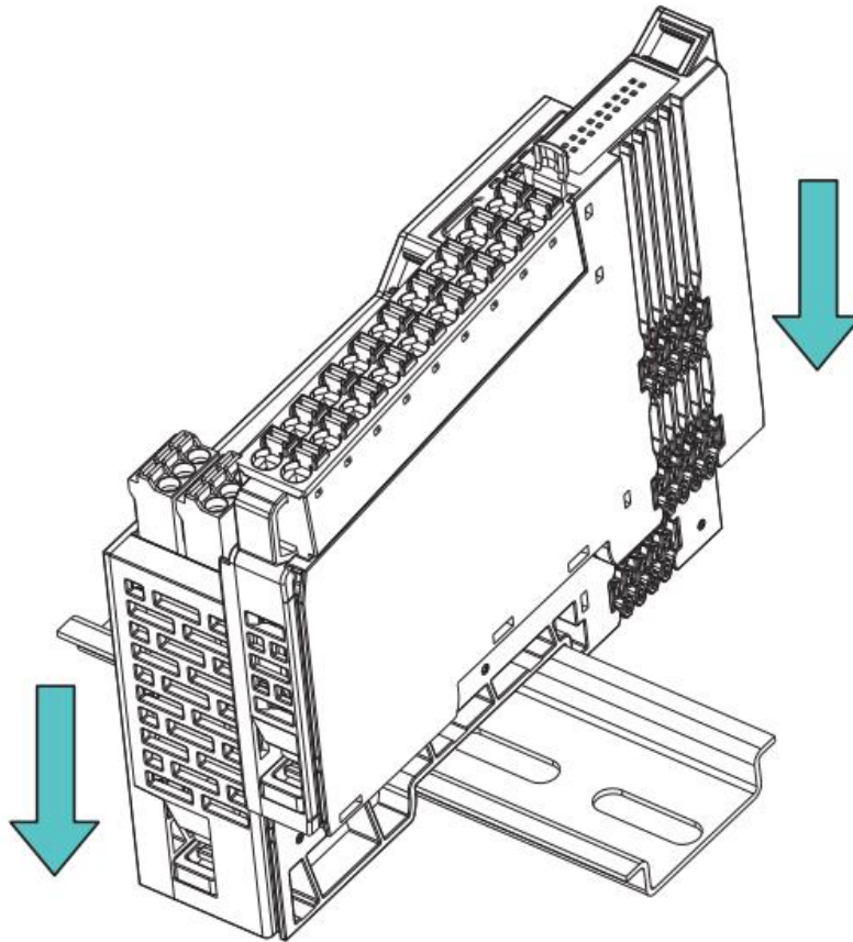
圖 6.1 模組安裝示意圖
