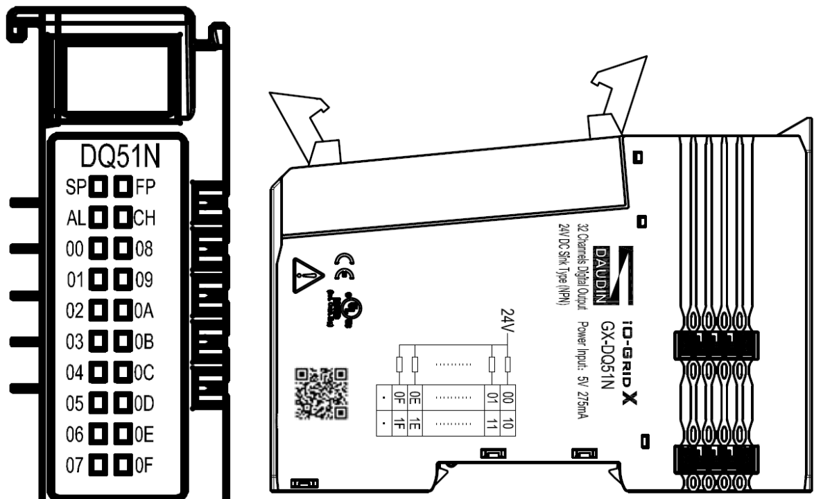
圖 4.15 GX-DQ51N 圖面
