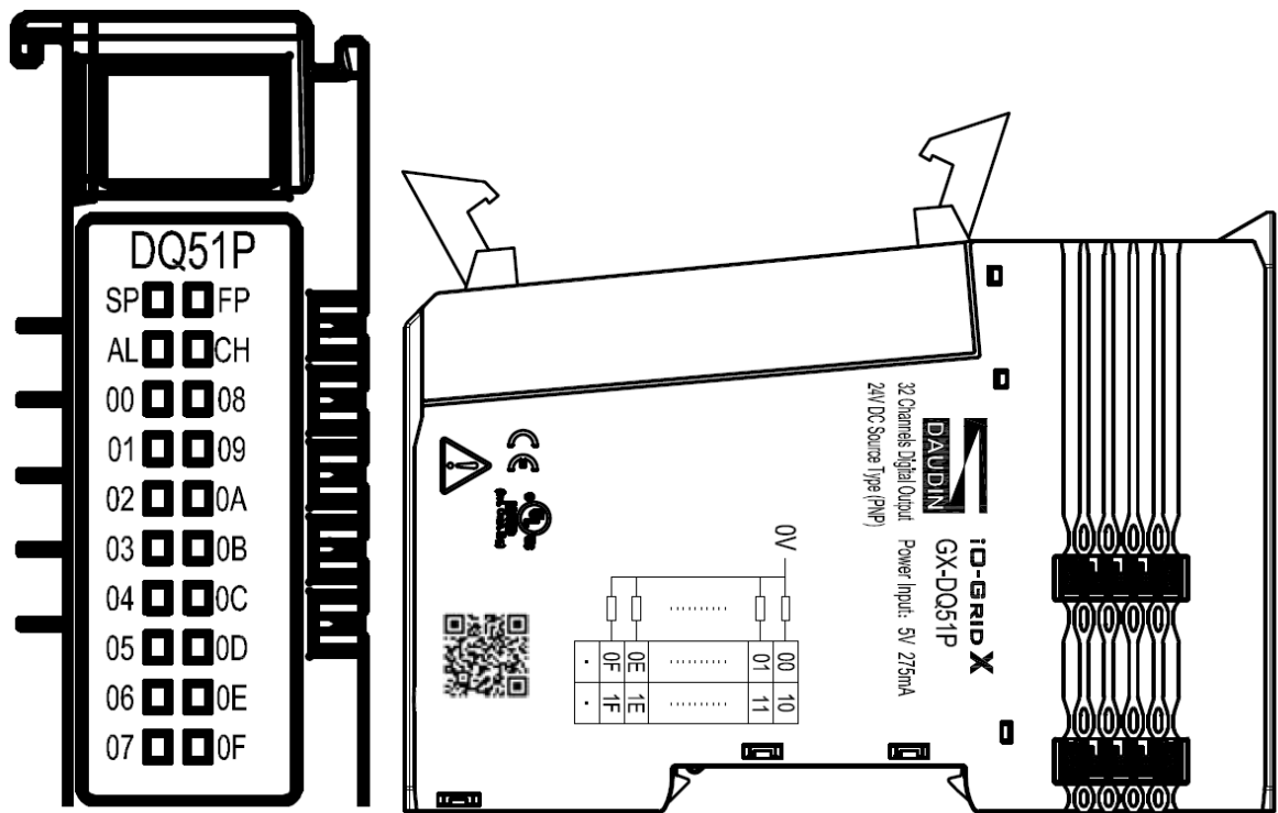
圖 4. 16 GX-DQ51P 圖面
