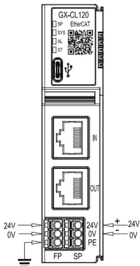
圖 8.1 耦合器接線圖
