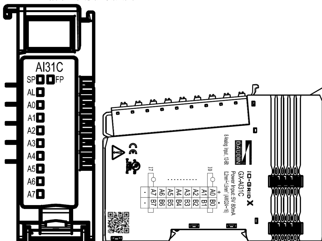
圖 4.22 GX-AI31C 圖面
